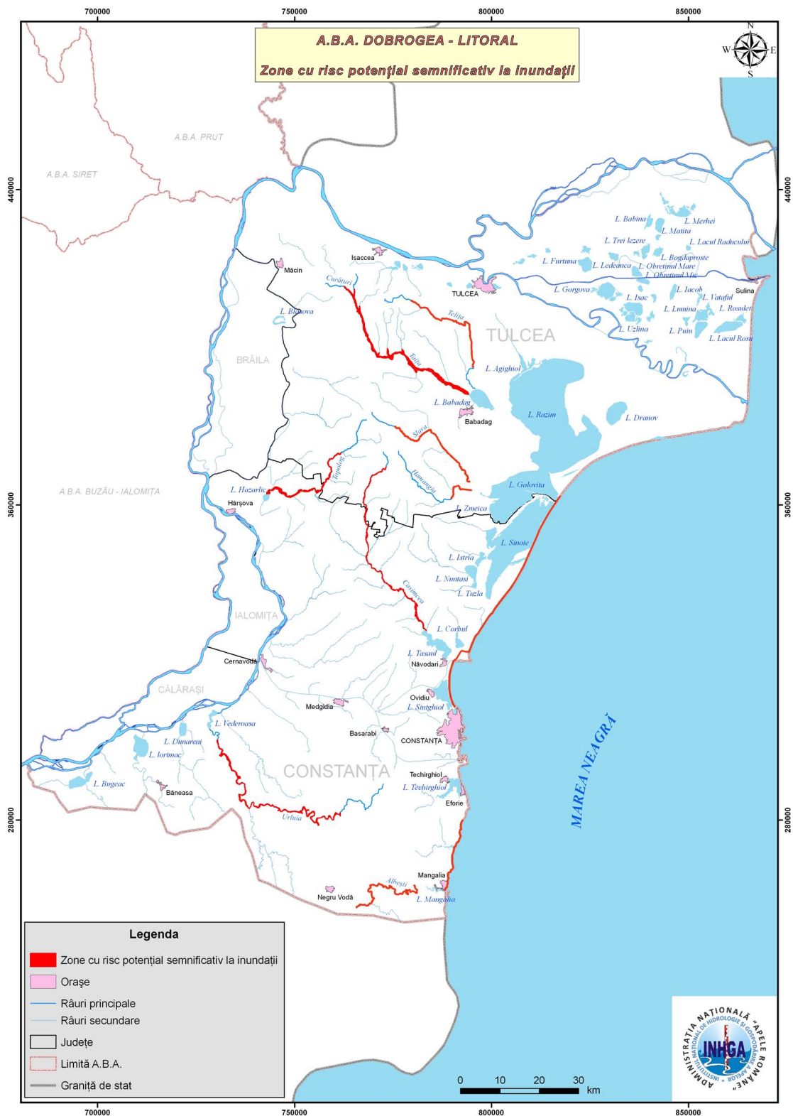
Figura 11 Localizarea zonelor cu risc potențial semnificativ la inundații identificate în cadrul Administrației Bazinale de Apă Dobrogea - Litoral
